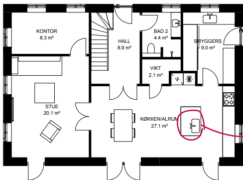
STUEPLAN 100 m 2
