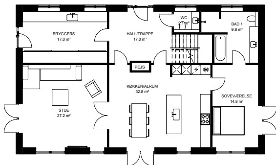
STUEPLAN 144,2 m 2
