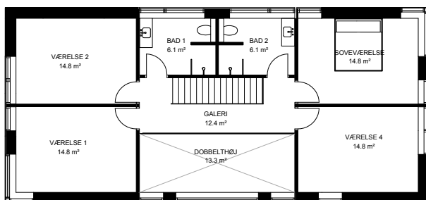
1. SALSPLAN 106 m 2
